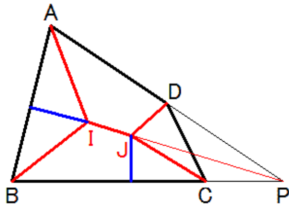
I = \triangle PAB の内心 J = \triangle CDP の傍心
