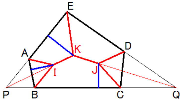
I = \triangle PAB の傍心 J = \triangle QCD の傍心 K = \triangle EPQ の内心
